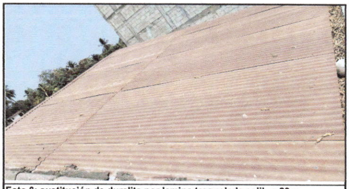
Foto 6: sustitución de duralita por lamina troquelada calibre 26 y mantenimiento de soporte de metal
