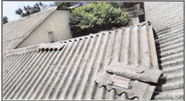
Foto 2: sustitución de duralita por lamina troquelada calibre 26 y mantenimiento de soporte de metal
